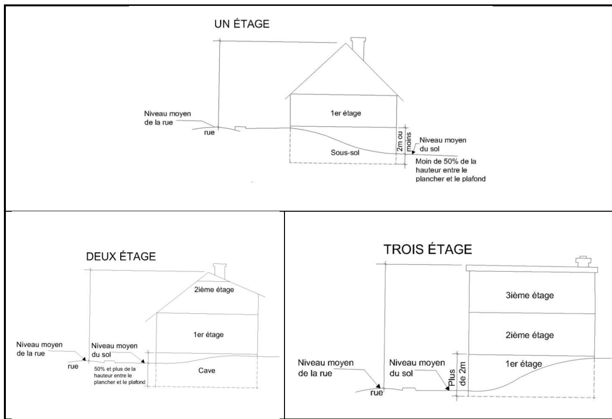
CROQUIS 7 : DETERMINATION DU NOMBRE D'ETAGE D'UN BATIMENT
